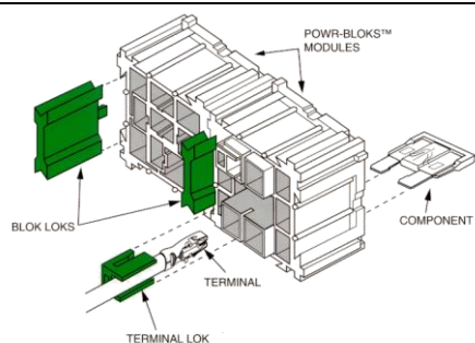
8354502 SÄKRINGS-BLOCK för 4 st ATO-Bladsäkringar
